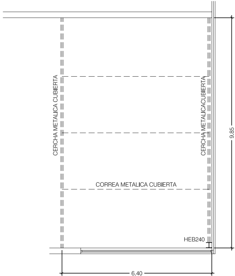
NAVE C (ESTADO ACTUAL)
